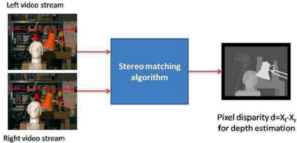
Şekil 8: Görsel görüntü eşleştirme algoritması gösterilmiştir.
