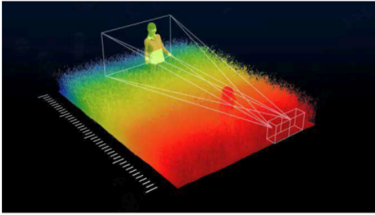
Şekil 10: Bu görselde, hesaplanan derinlik (Z) değerlerinin 2D düzlemde çıkarılarak 3D koordinat sistemine aktarılması görülmektedir. Renk skalası, nesnelerin kameraya olan mesafesini temsil eder. Kırmızı/sıcak bölgeler yakını, mavi/soğuk bölgeler ise uzağı simgeler.
